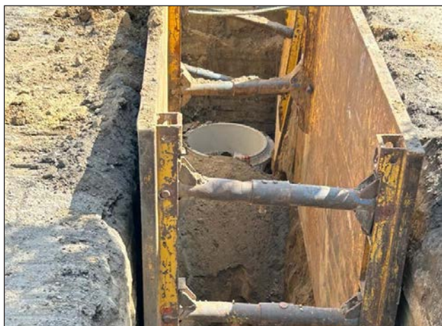
Budowa kanalizacji sanitarnej Zakrzewo ul. Polanki
